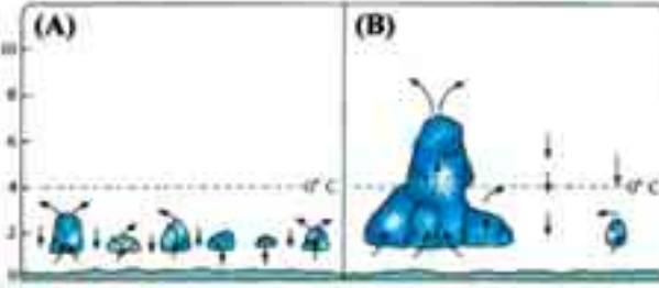
(A) Ayrı ayrı küçük bulut parçaları (kümülo-nimbüs bulutları) (B) Küçük bulutlar biraraya geldiğinde oluşan daha büyük bulutun içindeki yukarı çekilmeler artar, böylece bulutlar yukarıya doğru yığılır.
